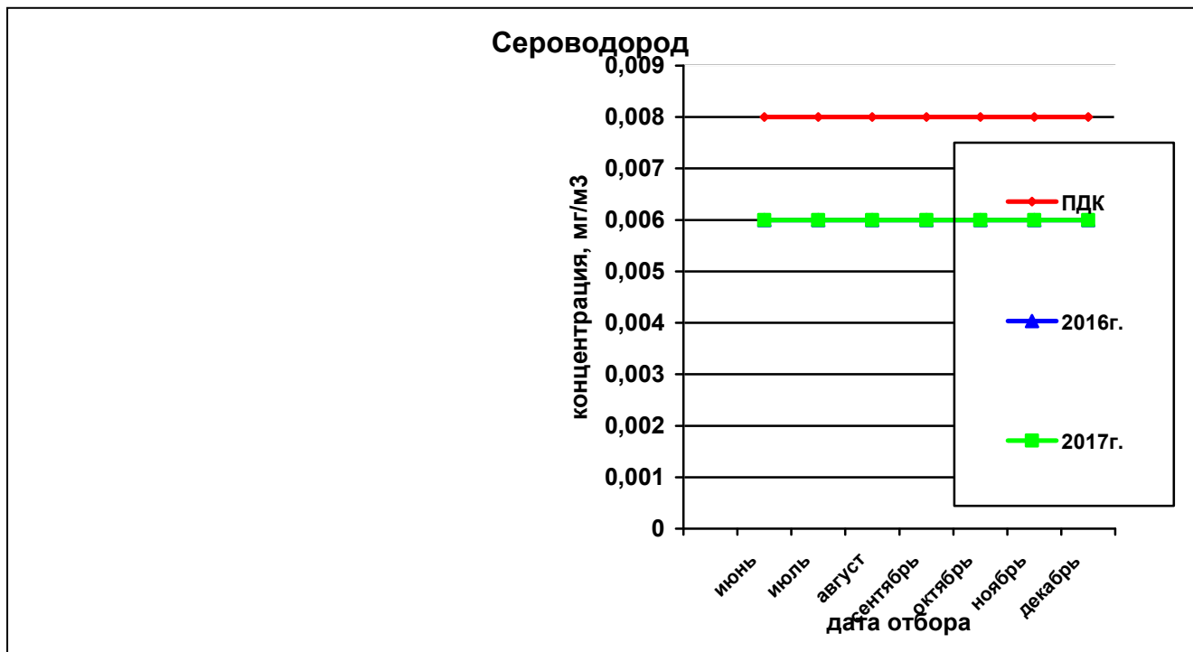
Рисунок 21— Сравнительная характеристика изменения концентрации сероводорода в атмосферном воздухе на ул. Костычева за 2016 и 2017гг.
