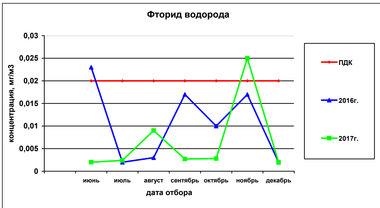
Рисунок 59— Сравнительная характеристика изменения концентрации фторида водорода в атмосферном воздухе у домов по ул. Вавилова, 21 – Малкова, 22 за 2016 и 2017гг.
