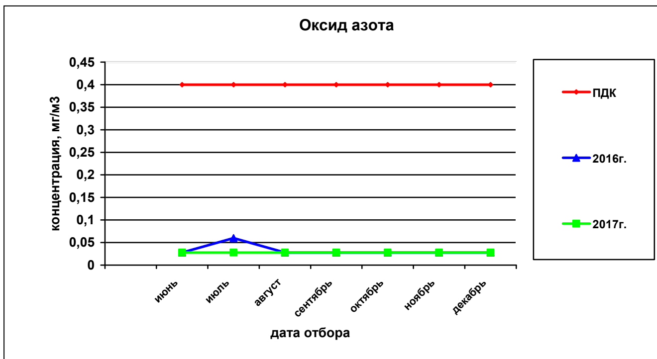
Рисунок 34— Сравнительная характеристика изменения концентрации оксида азота в атмосферном воздухе на ул. Строителей за 2016 и 2017гг.
