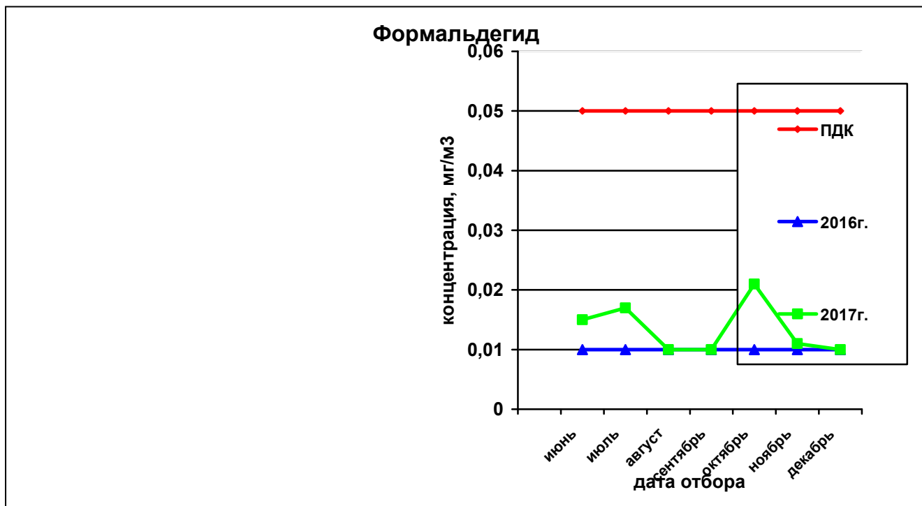
Рисунок 57— Сравнительная характеристика изменения концентрации формальдегида в атмосферном воздухе у домов по ул. Вавилова, 21 – Малкова, 22 за 2016 и 2017гг.
