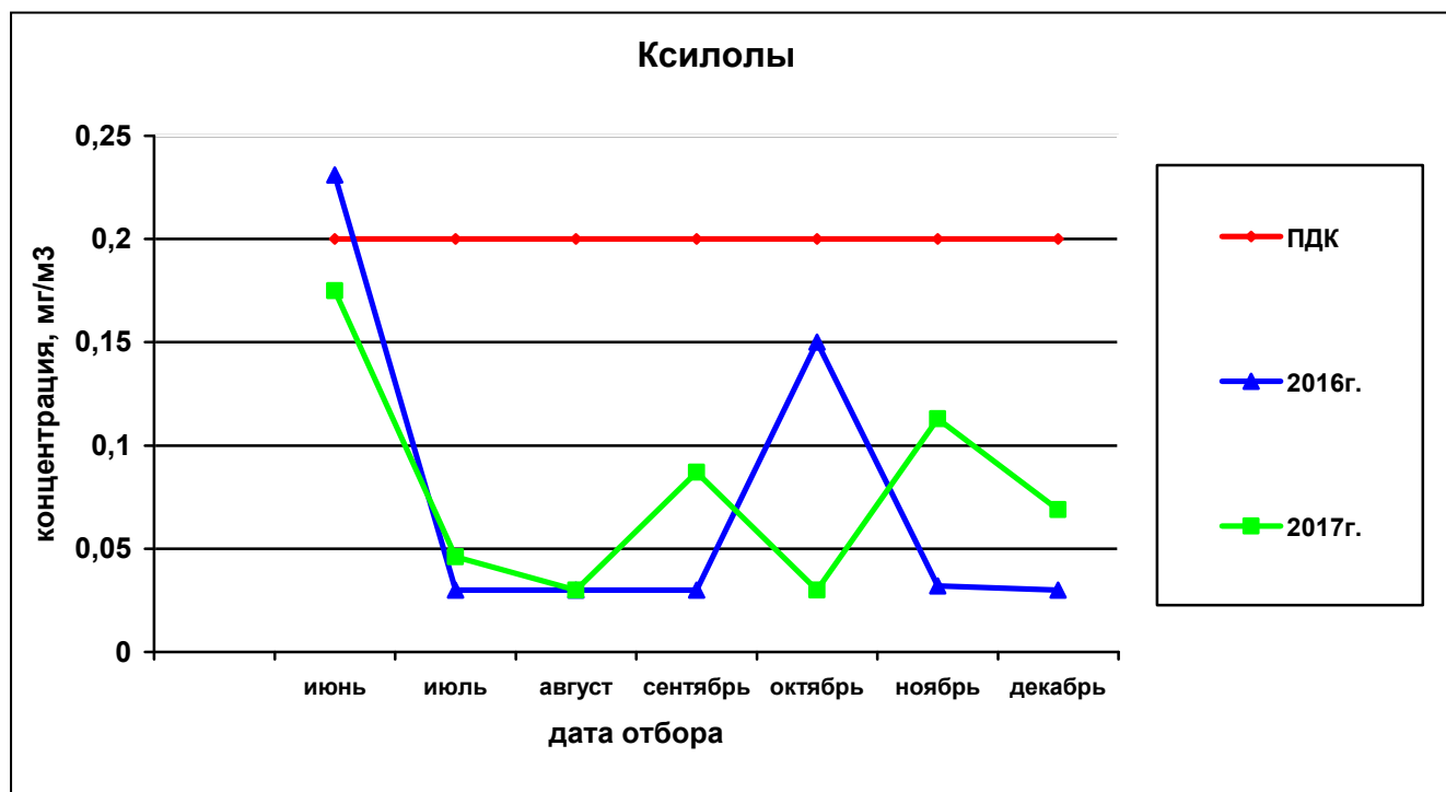
Рисунок 31— Сравнительная характеристика изменения концентрации ксилолов в атмосферном воздухе на ул. Костычева за 2016 и 2017гг.
