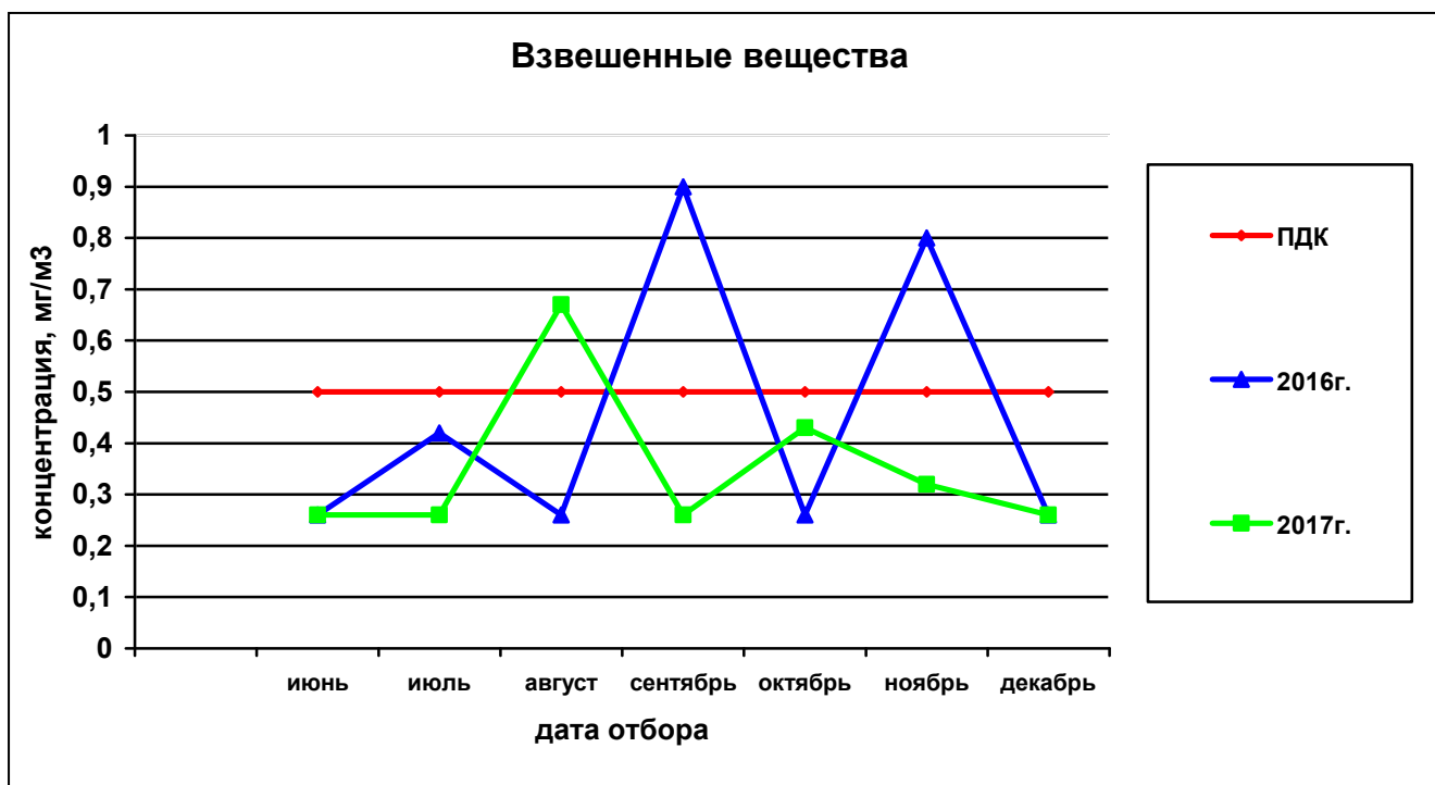
Рисунок 58— Сравнительная характеристика изменения концентрации взвешенных веществ в атмосферном воздухе у домов по ул. Вавилова, 21 – Малкова, 22 за 2016 и 2017гг.
