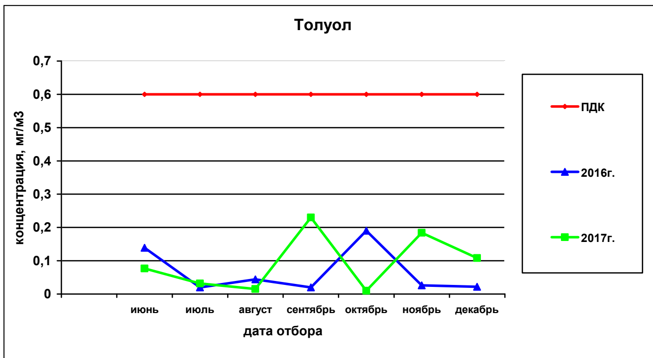
Рисунок 30— Сравнительная характеристика изменения концентрации толуола в атмосферном воздухе на ул. Костычева за 2016 и 2017гг.
