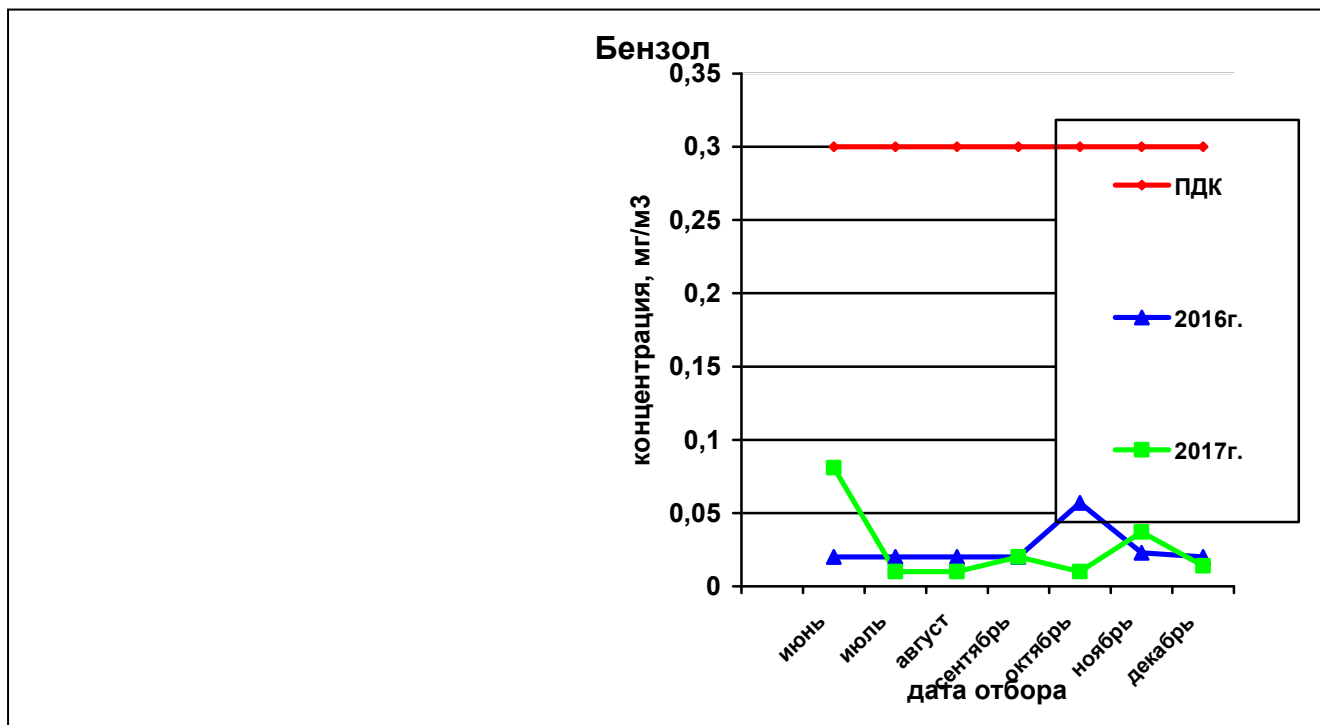
Рисунок 29— Сравнительная характеристика изменения концентрации бензола в атмосферном воздухе на ул. Костычева за 2016 и 2017гг.
