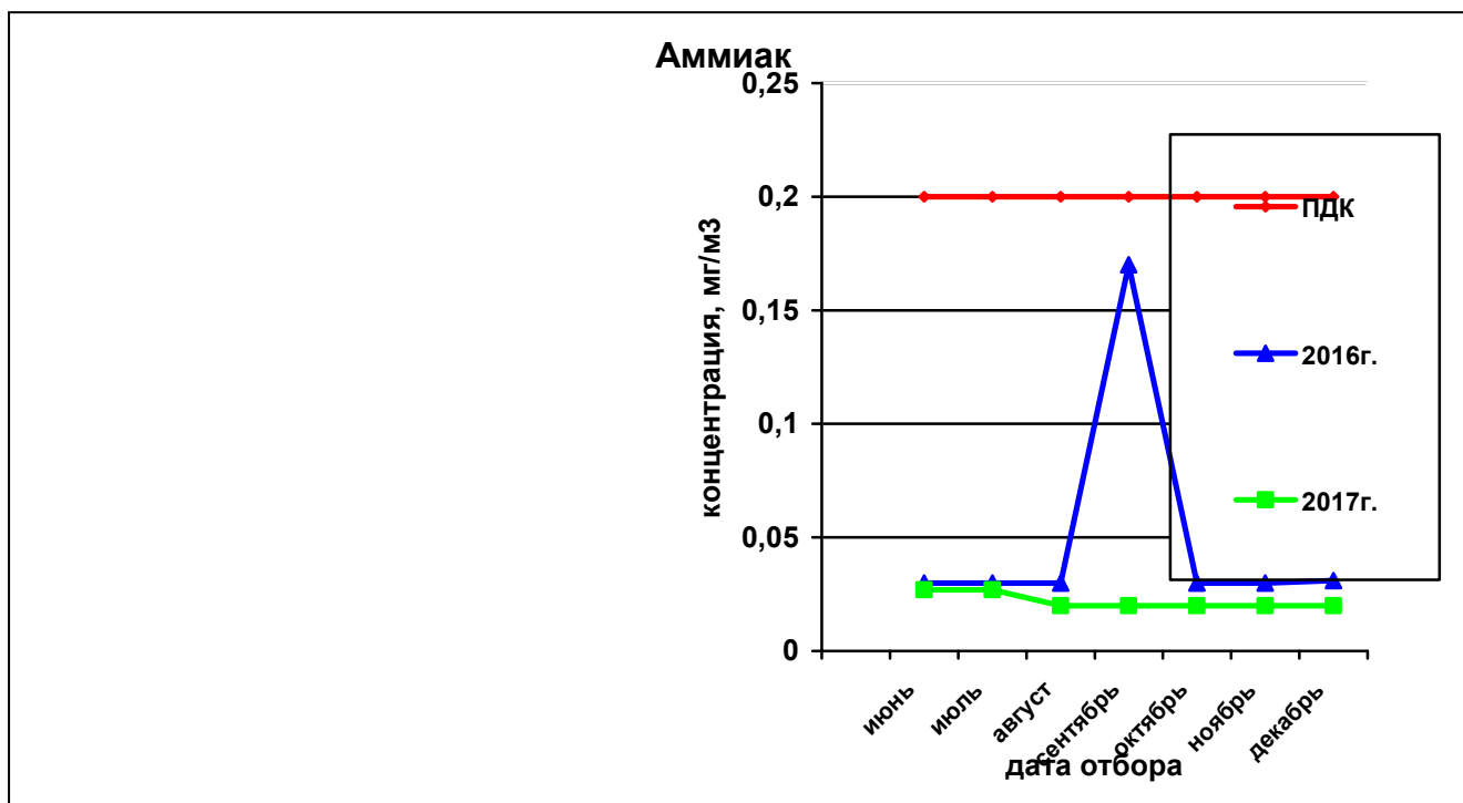
Рисунок 22— Сравнительная характеристика изменения концентрации аммиака в атмосферном воздухе на ул. Костычева за 2016 и 2017гг.
