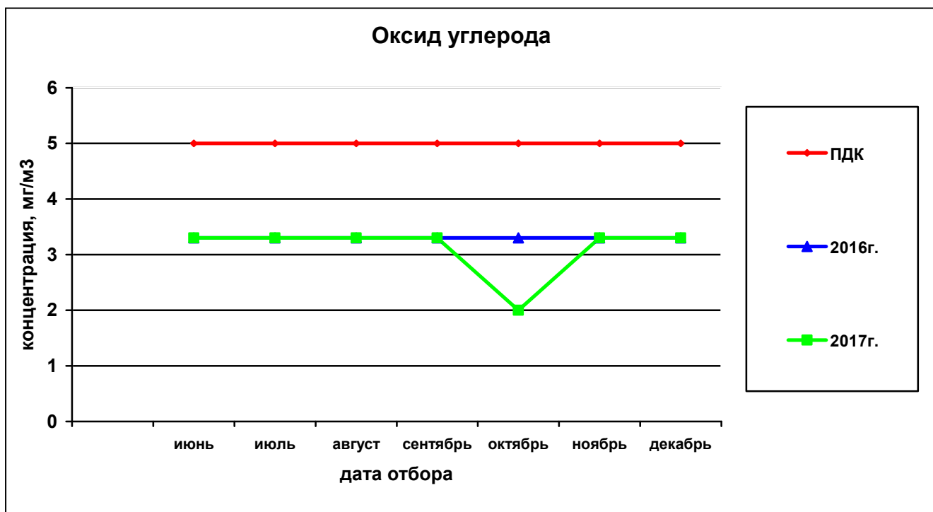
Рисунок 71— Сравнительная характеристика изменения концентрации оксида углерода в атмосферном воздухе на ул.Петропавловская,185 за 2016 и 2017гг.
