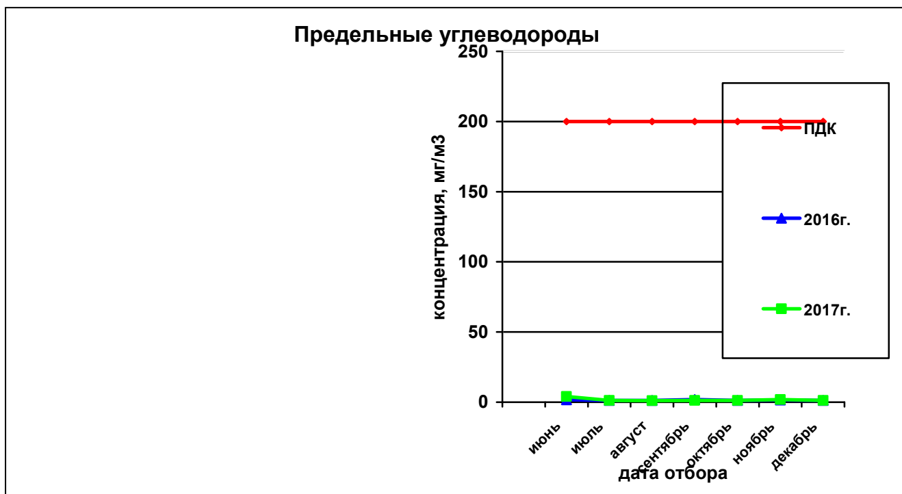
Рисунок 28— Сравнительная характеристика изменения концентрации предельных углеводородов в атмосферном воздухе на ул. Костычева за 2016 и 2017гг.
