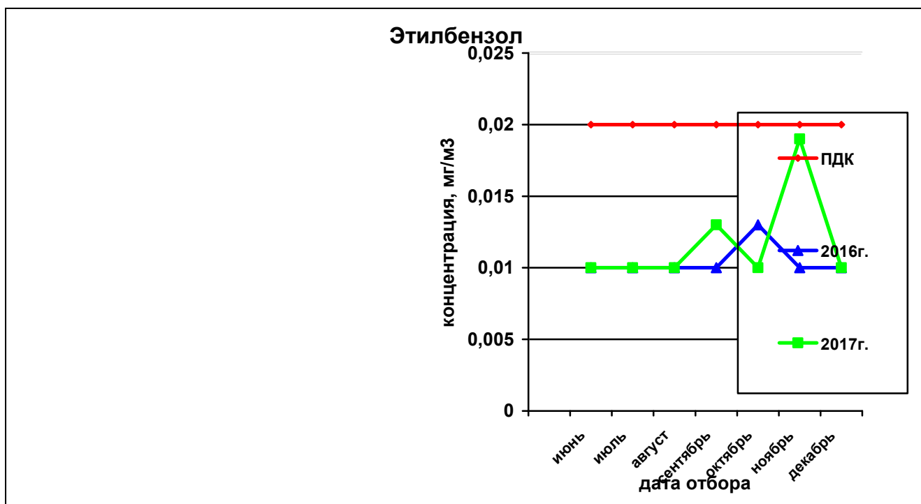
Рисунок 80— Сравнительная характеристика изменения концентрации этилбензола в атмосферном воздухе на ул.Петропавловская,185 за 2016 и 2017гг.
