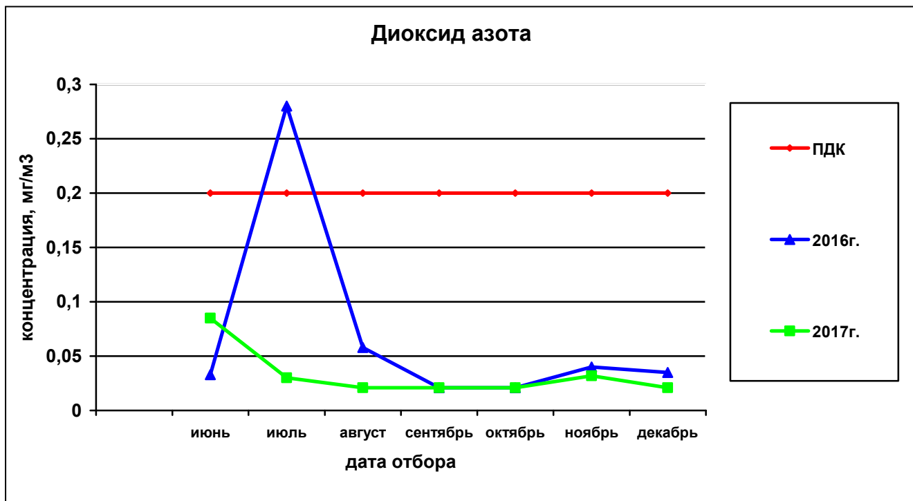
Рисунок 65— Сравнительная характеристика изменения концентрации диоксида азота в атмосферном воздухе на ул.Петропавловская,185 за 2016 и 2017гг.
