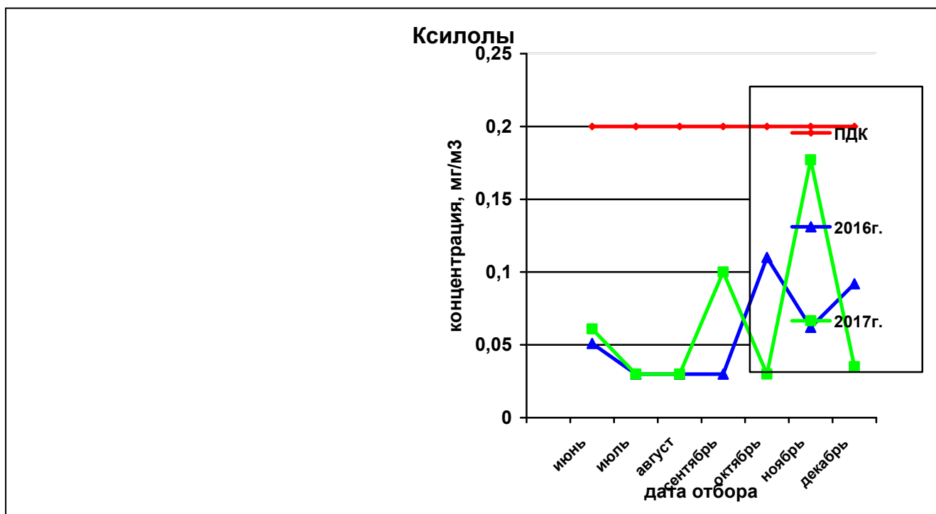
Рисунок 47— Сравнительная характеристика изменения концентрации ксилолов в атмосферном воздухе на ул. Строителей за 2016 и 2017гг.
