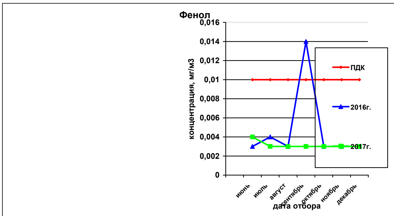
Рисунок 56— Сравнительная характеристика изменения концентрации фенола в атмосферном воздухе у домов по ул. Вавилова, 21 – Малкова, 22 за 2016 и 2017гг.
