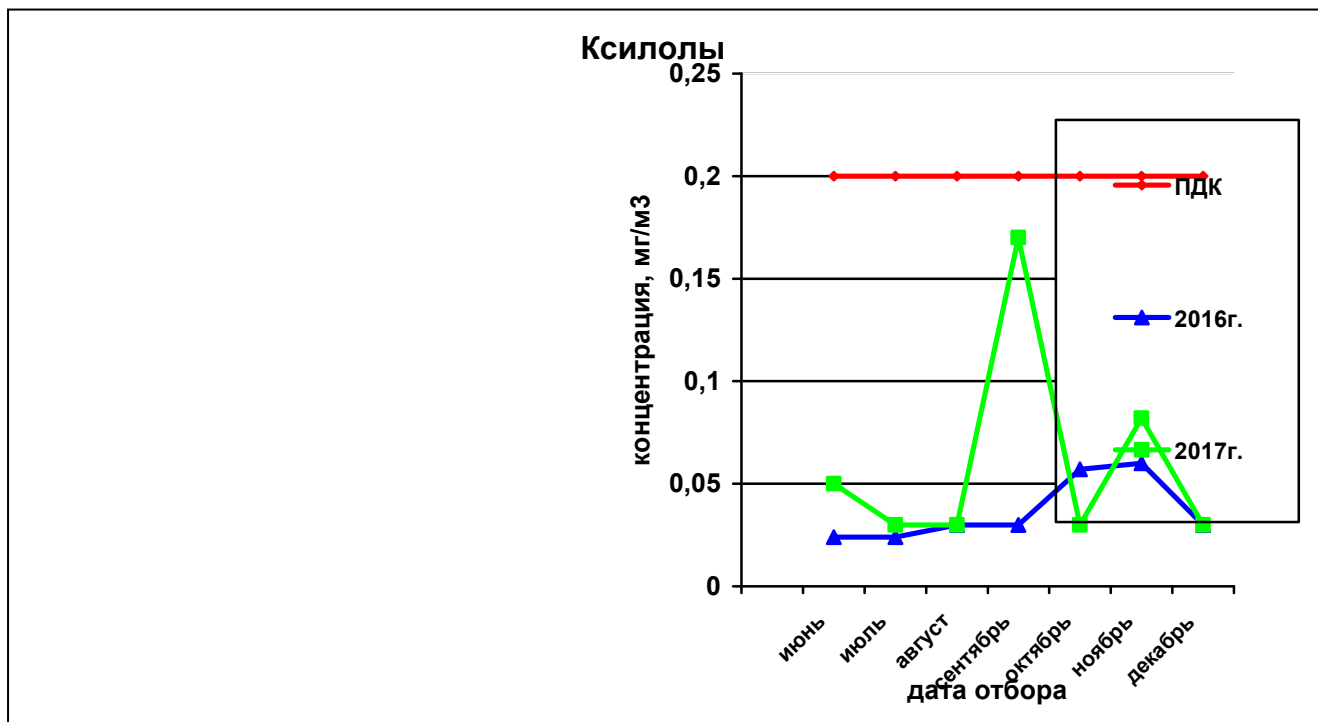
Рисунок 79— Сравнительная характеристика изменения концентрации ксилолов в атмосферном воздухе на ул.Петропавловская,185 за 2016 и 2017гг.
