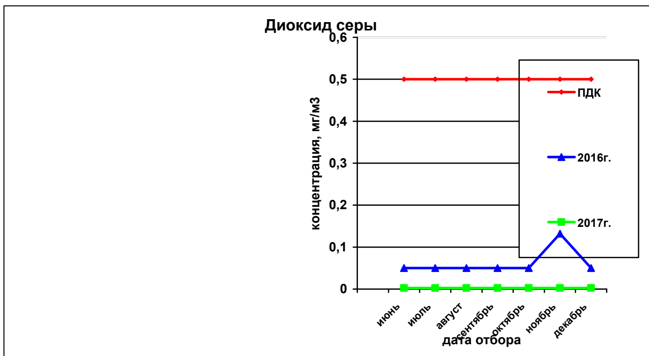
Рисунок 68— Сравнительная характеристика изменения концентрации диоксида серы в атмосферном воздухе на ул.Петропавловская,185 за 2016 и 2017гг.
