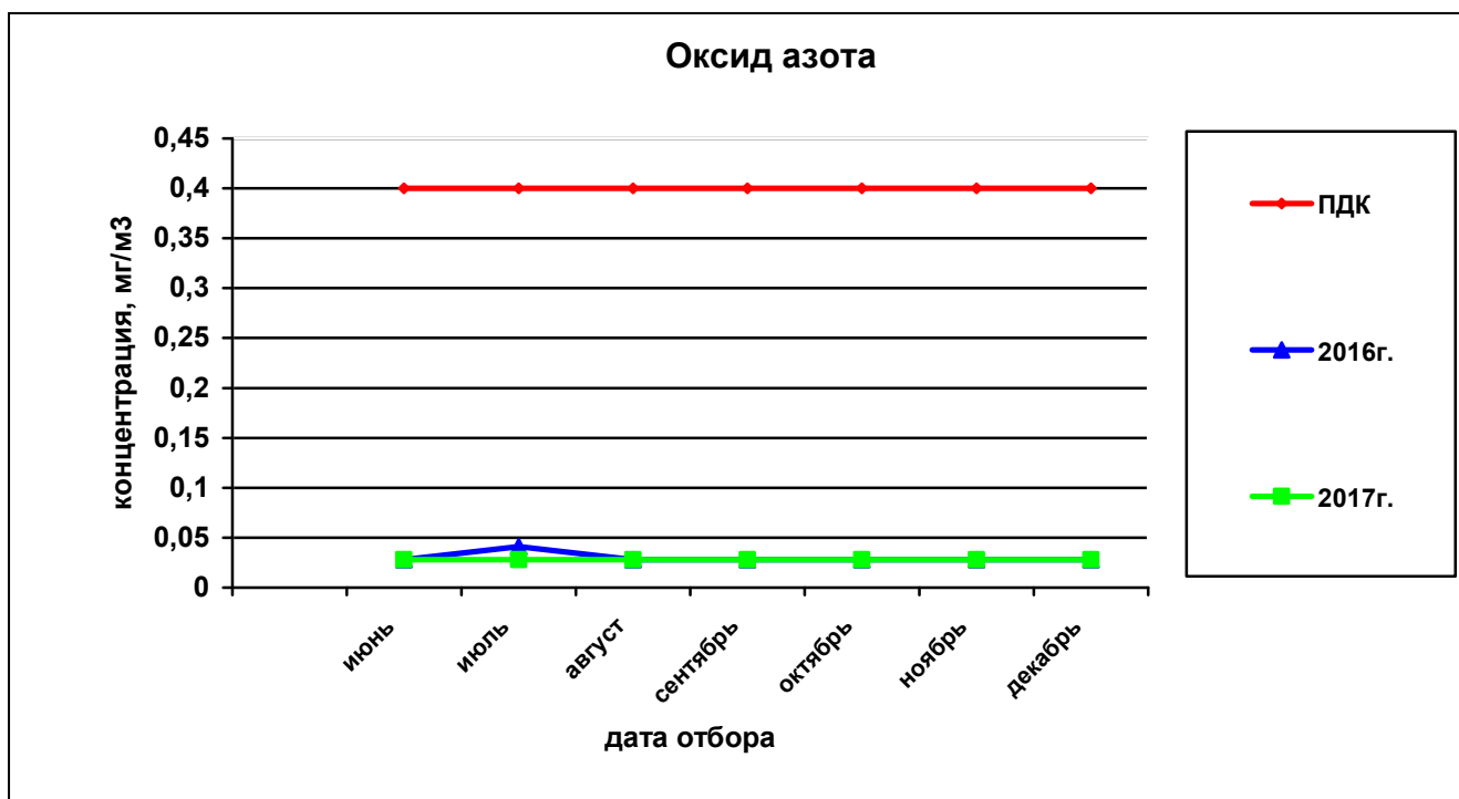
Рисунок 18— Сравнительная характеристика изменения концентрации оксида азота в атмосферном воздухе на ул. Костычева за 2016 и 2017гг.
