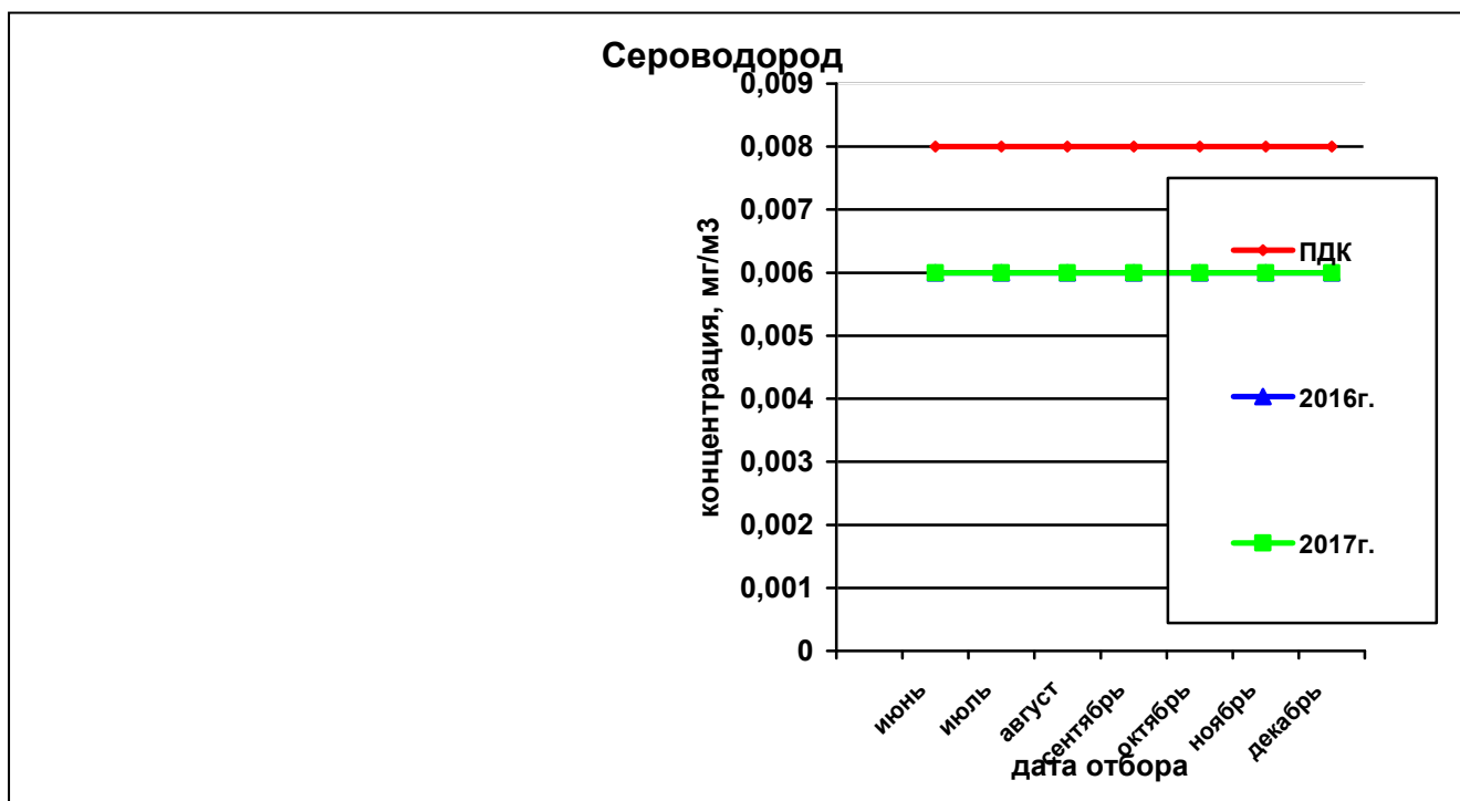
Рисунок 53— Сравнительная характеристика изменения концентрации сероводорода в атмосферном воздухе у домов по ул. Вавилова, 21 – Малкова, 22 за 2016 и 2017гг.
