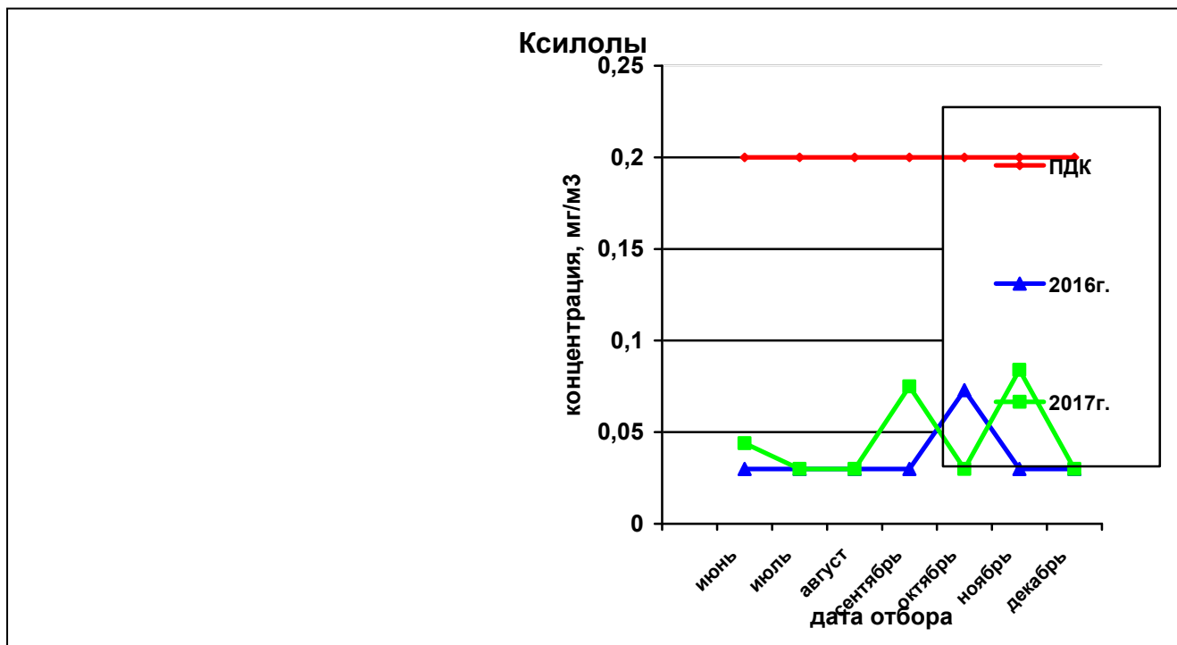
Рисунок 63— Сравнительная характеристика изменения концентрации ксилолов в атмосферном воздухе у домов по ул. Вавилова, 21 – Малкова, 22 за 2016 и 2017гг.
