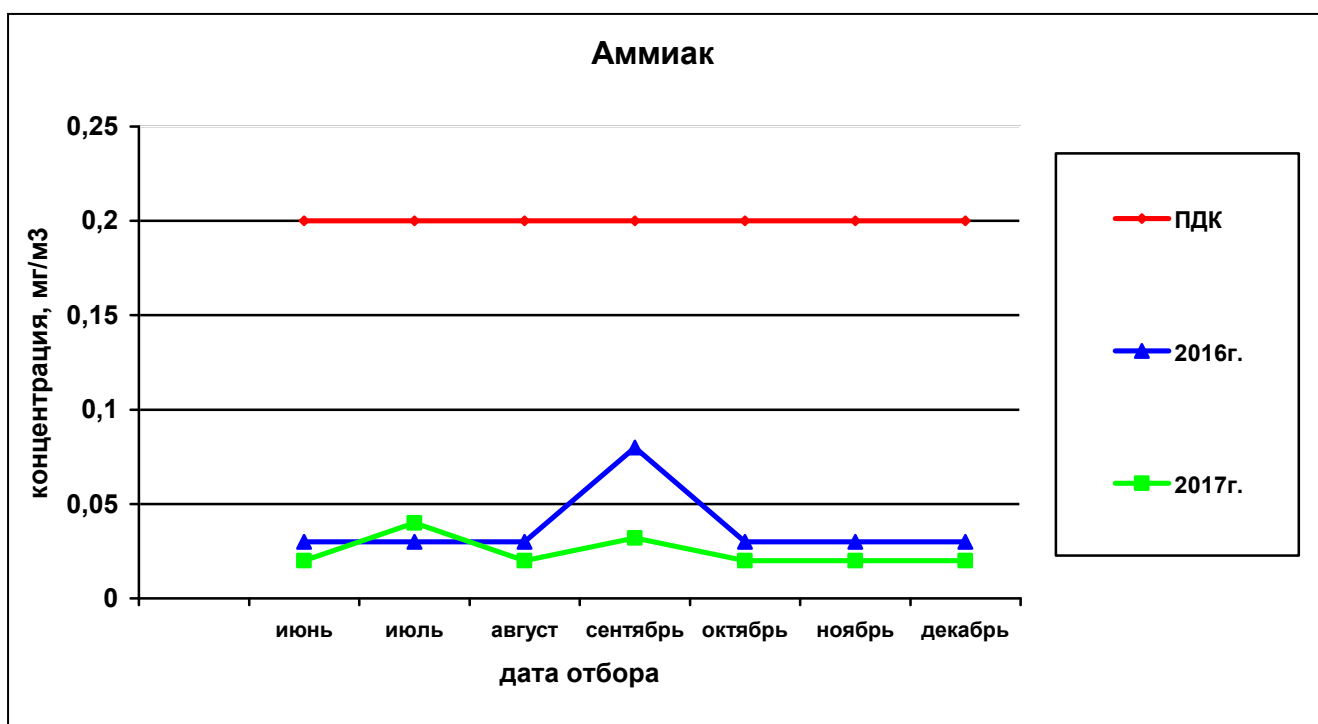
Рисунок 70— Сравнительная характеристика изменения концентрации аммиака в атмосферном воздухе на ул.Петропавловская,185 за 2016 и 2017гг.
