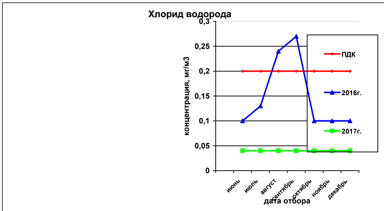
Рисунок 51— Сравнительная характеристика изменения концентрации хлорида водорода в атмосферном воздухе у домов по ул. Вавилова, 21 – Малкова, 22 за 2016 и 2017гг.
