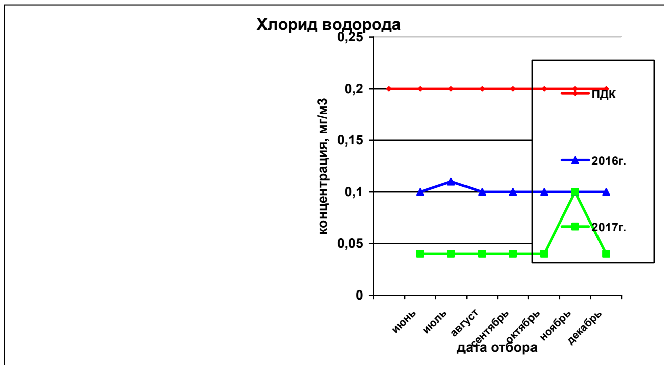
Рисунок 35— Сравнительная характеристика изменения концентрации хлорида водорода в атмосферном воздухе на ул. Строителей за 2016 и 2017гг.
