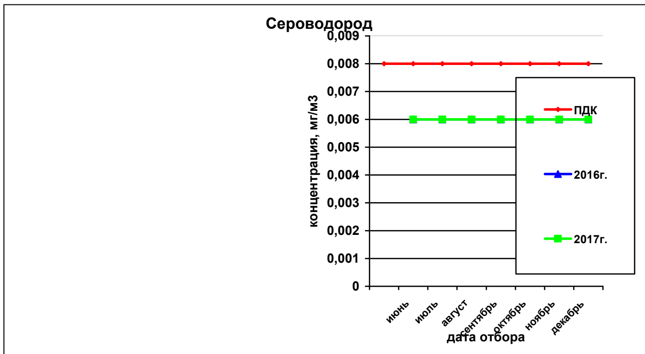
Рисунок 37— Сравнительная характеристика изменения концентрации сероводорода в атмосферном воздухе на ул. Строителей за 2016 и 2017гг.
