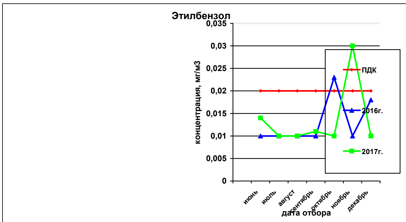
Рисунок 48— Сравнительная характеристика изменения концентрации этилбензола в атмосферном воздухе на ул. Строителей за 2016 и 2017гг.
