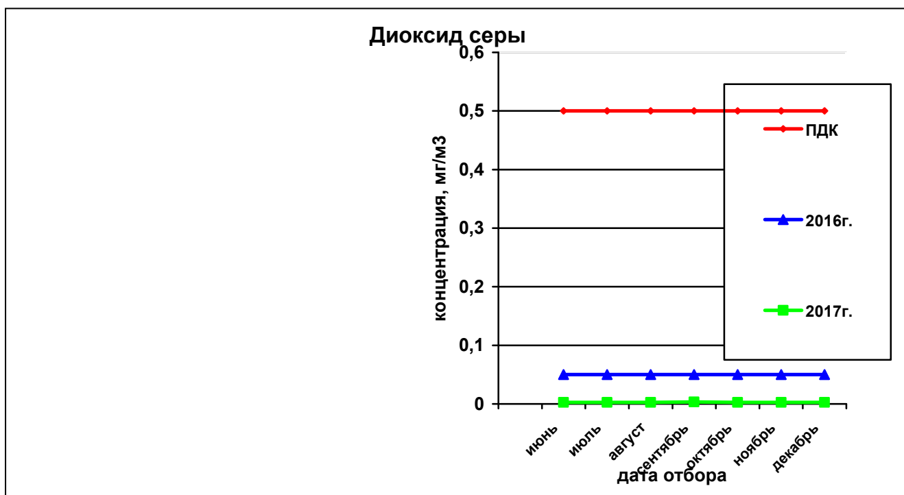
Рисунок 20— Сравнительная характеристика изменения концентрации диоксида серы в атмосферном воздухе на ул. Костычева за 2016 и 2017гг.
