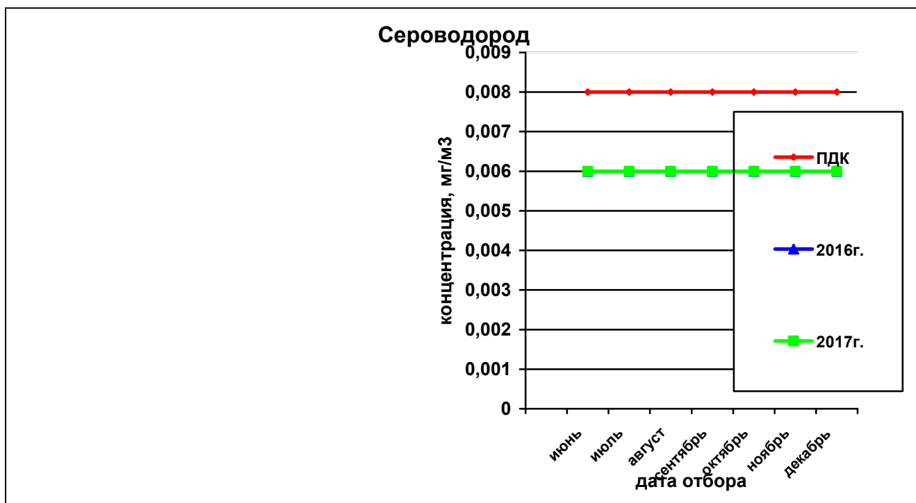
Рисунок 69— Сравнительная характеристика изменения концентрации сероводорода в атмосферном воздухе на ул.Петропавловская,185 за 2016 и 2017гг.
