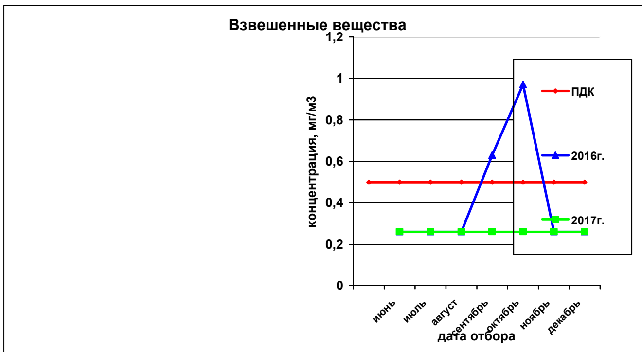
Рисунок 42— Сравнительная характеристика изменения концентрации взвешенных веществ в атмосферном воздухе на ул. Строителей за 2016 и 2017гг.
