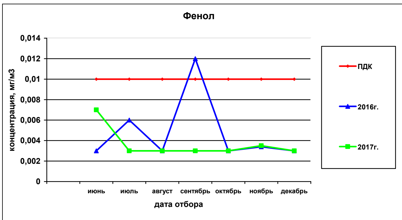
Рисунок 72— Сравнительная характеристика изменения концентрации фенола в атмосферном воздухе на ул.Петропавловская,185 за 2016 и 2017гг.
