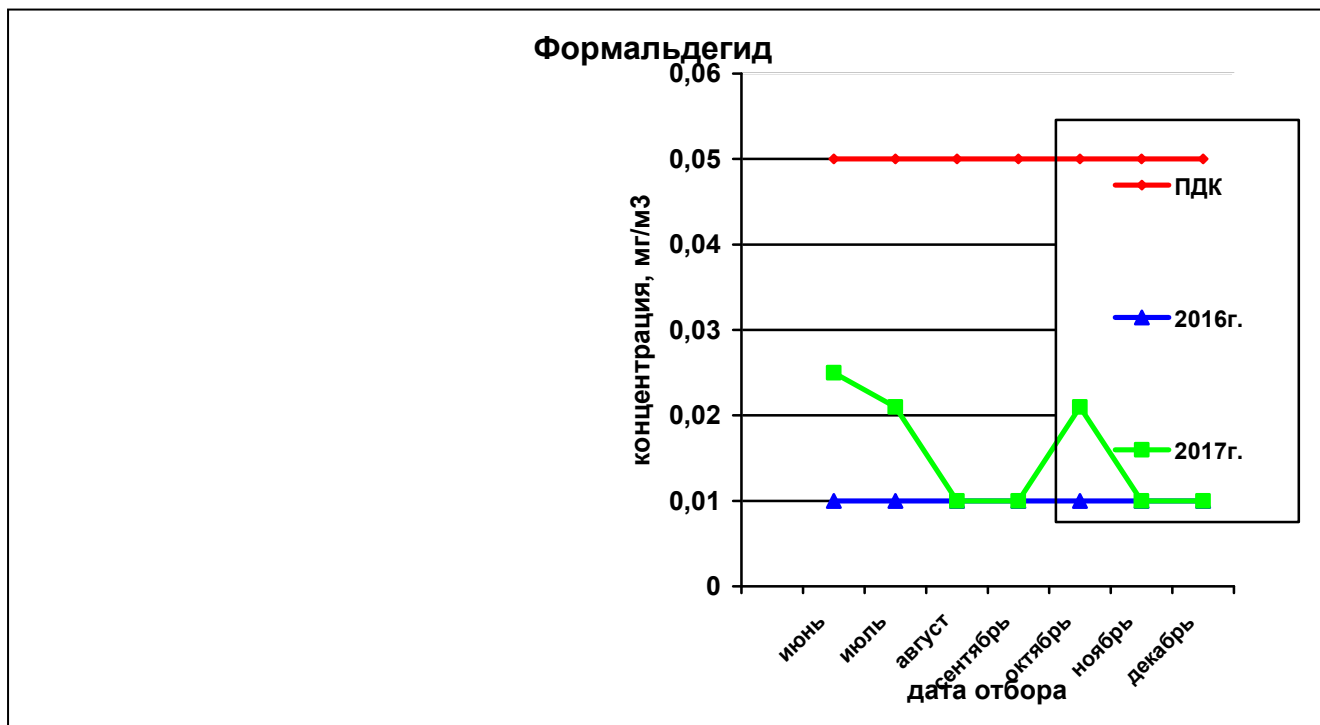
Рисунок 41— Сравнительная характеристика изменения концентрации формальдегида в атмосферном воздухе на ул. Строителей за 2016 и 2017гг.
