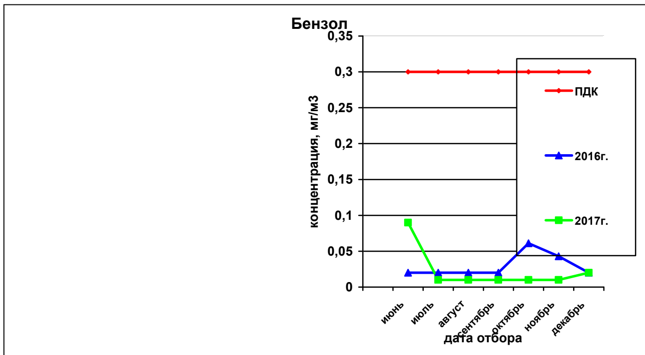
Рисунок 45— Сравнительная характеристика изменения концентрации бензола в атмосферном воздухе на ул. Строителей за 2016 и 2017гг.
