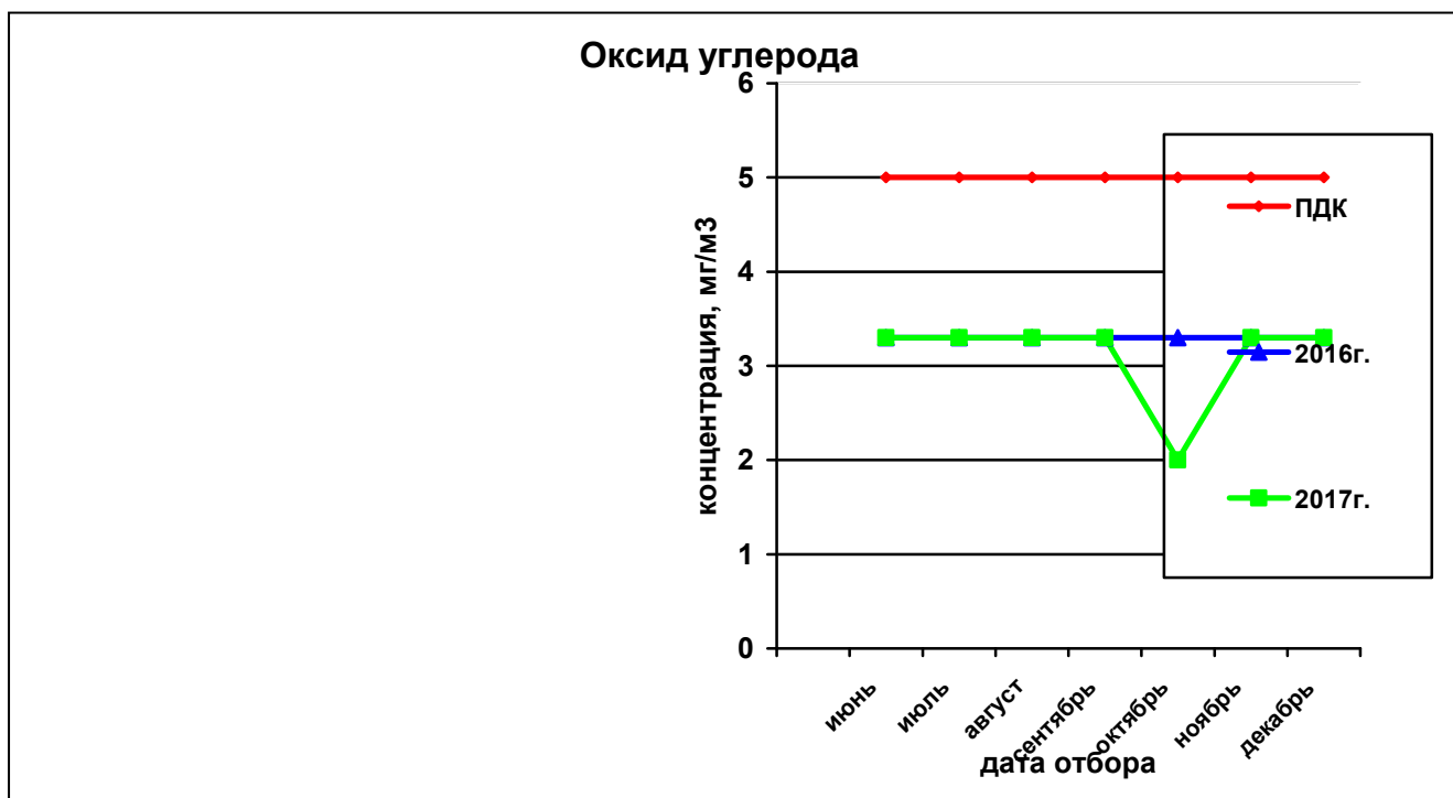
Рисунок 39— Сравнительная характеристика изменения концентрации оксида углерода в атмосферном воздухе на ул. Строителей за 2016 и 2017гг.
