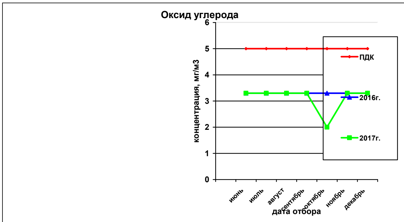
Рисунок 23— Сравнительная характеристика изменения концентрации оксида углерода в атмосферном воздухе на ул. Костычева за 2016 и 2017гг.
