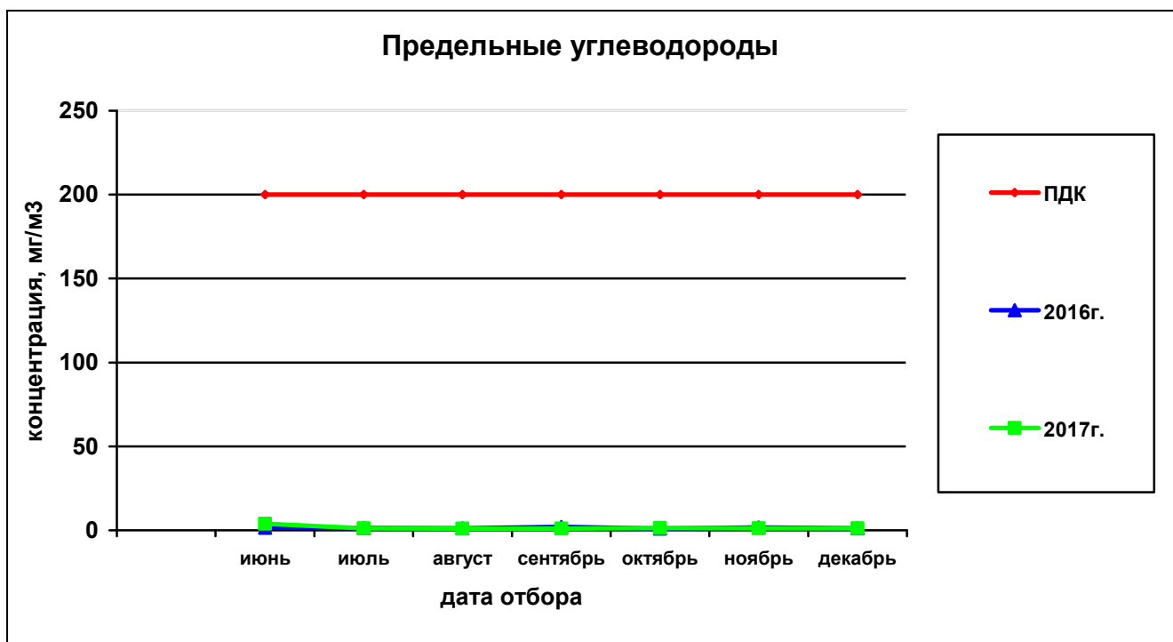
Рисунок 76— Сравнительная характеристика изменения концентрации предельных углеводородов в атмосферном воздухе на ул.Петропавловская,185 за 2016 и 2017гг.
