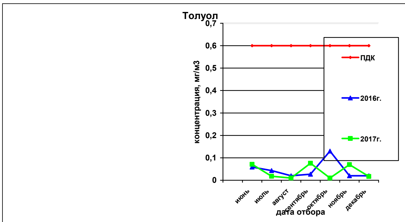
Рисунок 62— Сравнительная характеристика изменения концентрации толуола в атмосферном воздухе у домов по ул. Вавилова, 21 – Малкова, 22 за 2016 и 2017гг.
