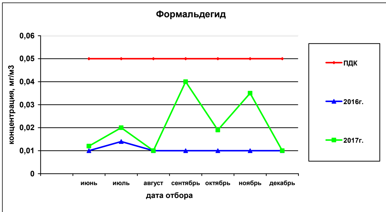
Рисунок 25— Сравнительная характеристика изменения концентрации формальдегида в атмосферном воздухе на ул. Костычева за 2016 и 2017гг.
