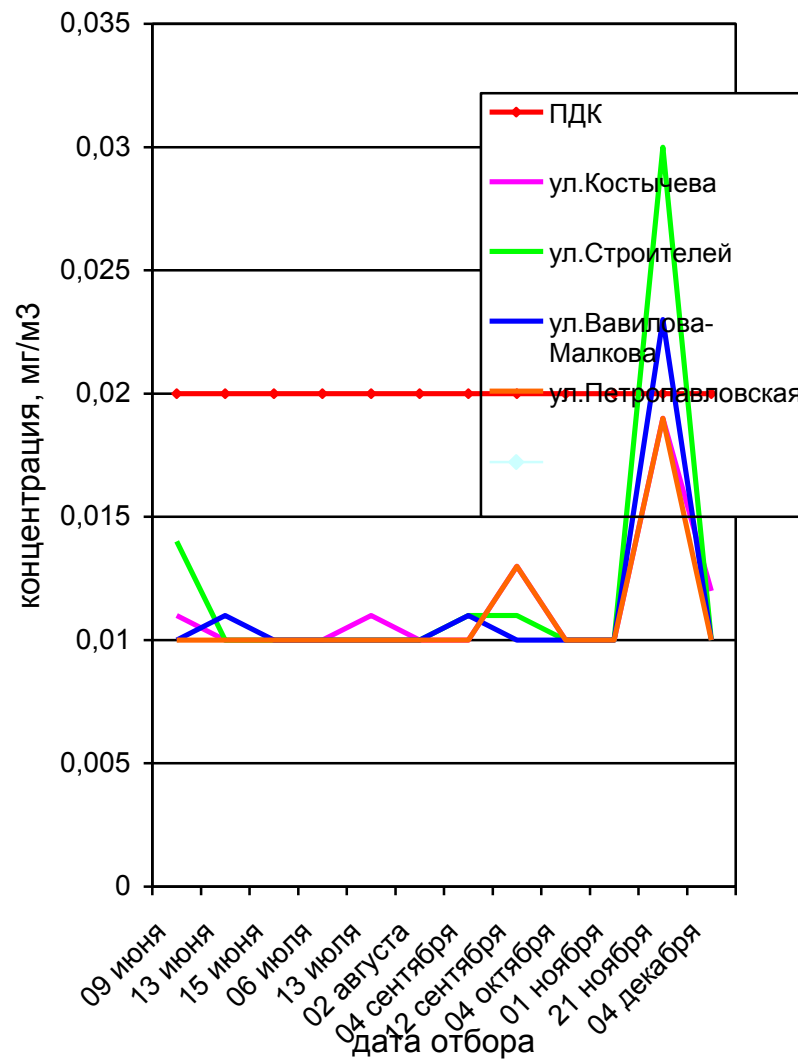
Рисунок 16 –Изменение концентрации этилбензола в атмосферном воздухе Дзержинского района г. Перми в 2017г.
